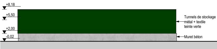
FACADE EST
