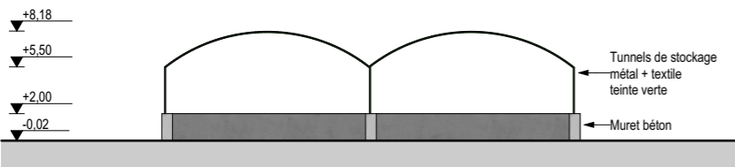
FACADE NORD
