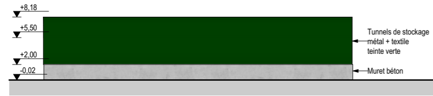
FACADE NORD
