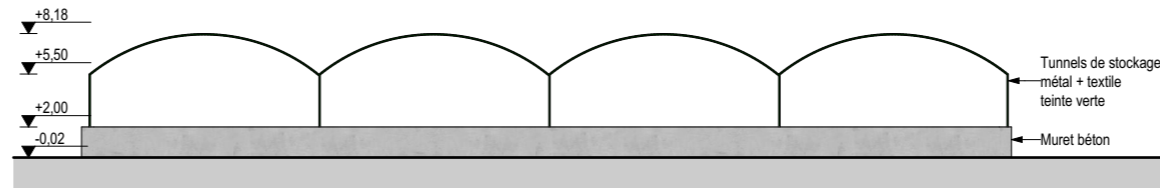
FACADE OUEST
